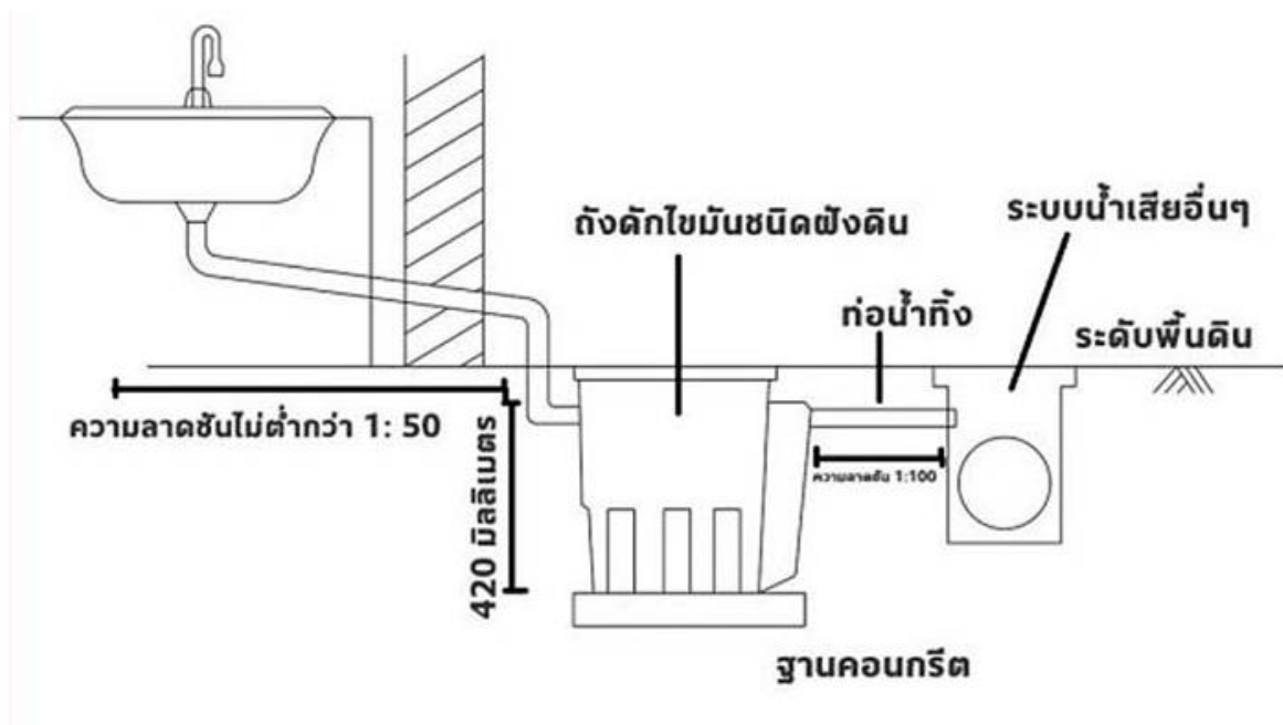
ภาพการติดตั้งถังดักไขมัน แบบฝังดินขนาดเล็ก
