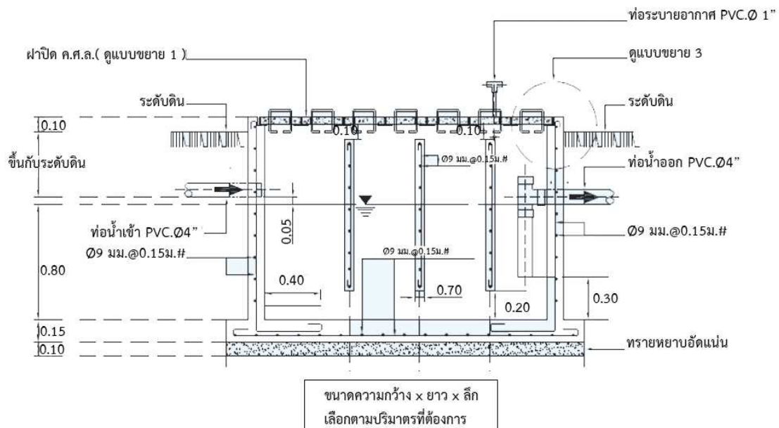
แปลนภาพตัดขวางของบ่อตกไขมัน แบบคอนกรีตเสริมเหล็ก
