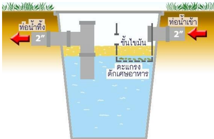
ถังดักไขมันฝังพื้นขนาดเล็ก
