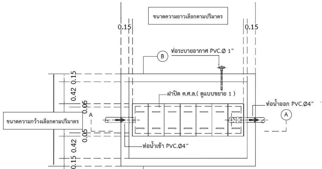
แปลนภาพด้านบนของบ่อตกไขมันแบบคอนกรีตเสริมเหล็ก
